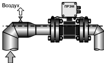
Рисунок 9 – Установка ПРЭМ в верхней точке трубопровода
