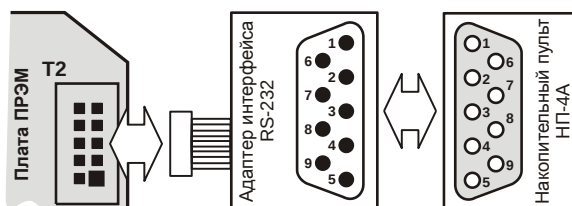
Рисунок И.2 – Схема подключения к НП-4А через внешний интерфейс RS-232
