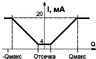
Рис. 5 – Выходная характеристика токового выхода ПРЭМ
