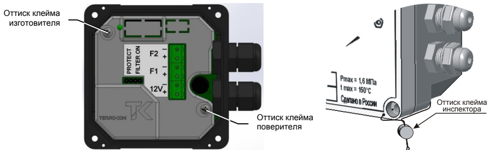
Рис. 4 – Места пломбирования
