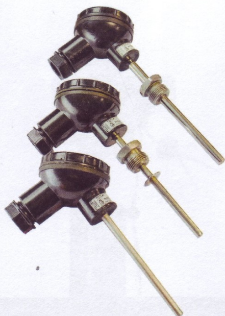
Рисунок 3 - Общий вид ТС исполнения 3 (головка типа DL)
