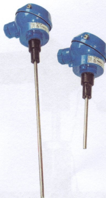
Рисунок 4 - Общий вид ТС исполнения 5 (головка типа PL)
