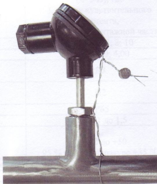
Рисунок 8 - Схема пломбировки ТС (головка типа DL)
