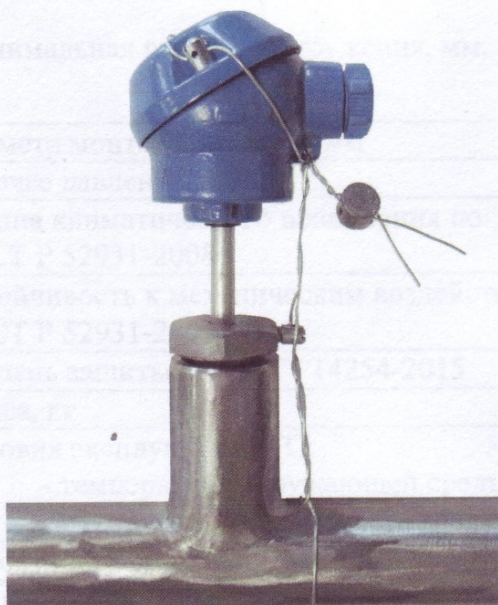
Рисунок 7 - Схема пломбировки ТС (головка типа PL)
